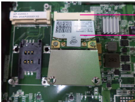
Mini PCIe slot
